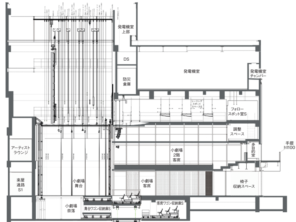
舞台断面図
