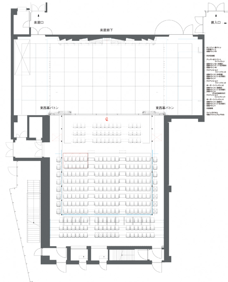
舞台平面図
