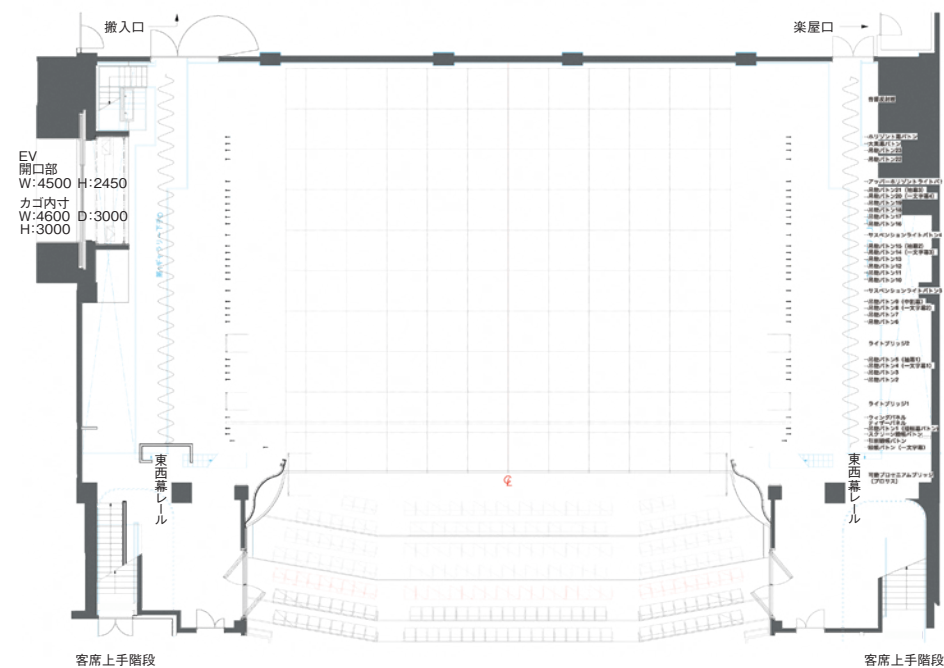
舞台平面図
